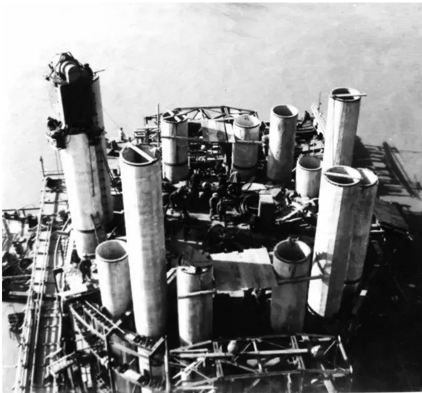
武汉长江大桥大型管柱施工现场
